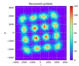
(c) 16-QAM.
